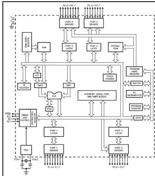
Gambar 2.1 Struktur Mikrokontroler ATmega 16
