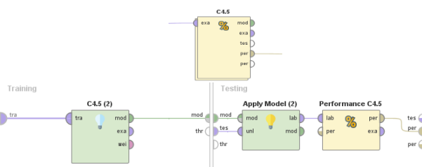
Gambar 3 Konfigurasi Model Algoritma C4.5
