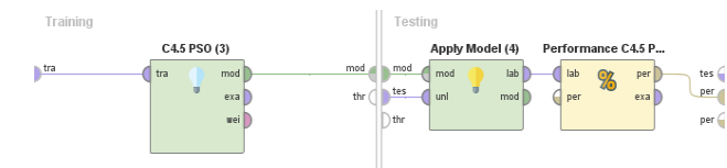
Gambar 11 Konfigurasi Algoritma C4.5 + PSO
