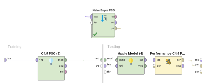
Gambar 15 Konfigurasi Model Algoritma Naïve Bayes PSO
