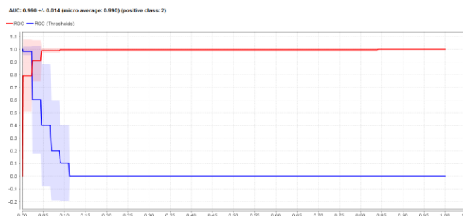
Gambar 10 Kurva ROC Algoritma Naïve Bayes
