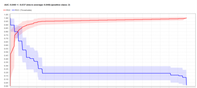
Gambar 6 Kurva ROC Algoritma C4.5
