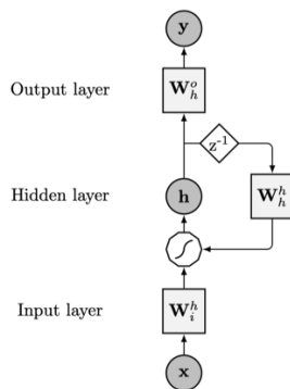
Gambar 1. Arsitektur RNN [7]
